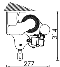
Montaggio a soffitto con staffa estrusa Ceiling installation with extruded bracket
