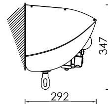
Montaggio con tettuccio Installation with a hood
